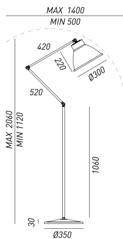
269.06.OF 1x Max 46W E27
