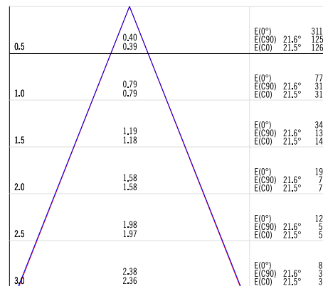
7W 40°
