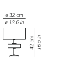
LSH04 --- Lampada da tavolo piccola Small table lamp 1xE27 70W HS CE IP20 □
