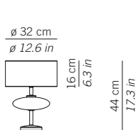
LSH03 --- Lampada da tavolo piccola Small table lamp 1xE27 70W HS CE IP20 □
